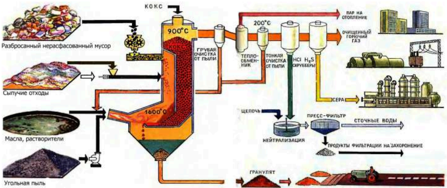
Схема работы завода
